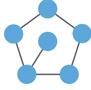
Sparse
