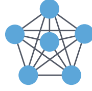
Dense
